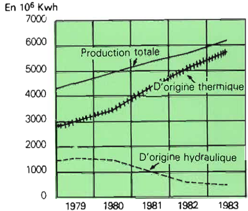
Production de l'énergie électrique
